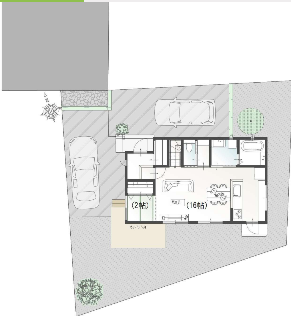
外構付1階平面
