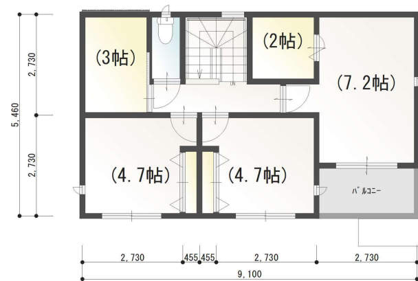
2階平面
